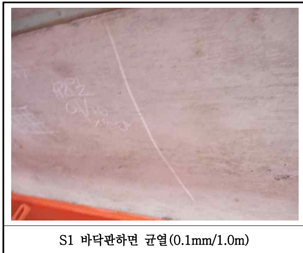
【사진 22.3.3】 바닥판하면 손상현황
