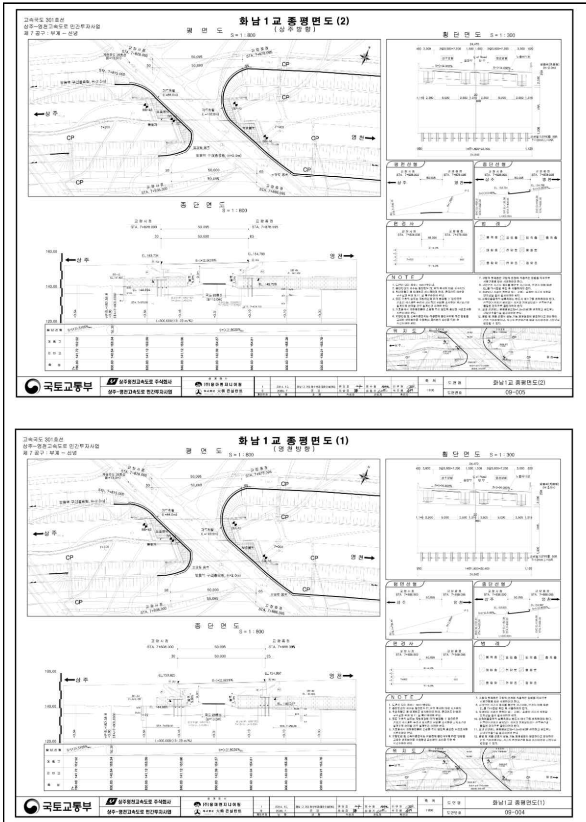
【그림 22.1.3】 종평면도
