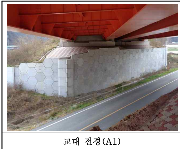
【사진 22.3.29】 교대 전경
