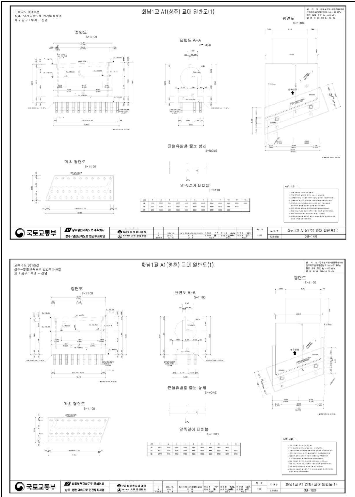
【그림 22.1.6】 교대 일반도
